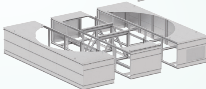
Separatori di gocce ad alta efficienza (Brevetto US 6.315.804)
